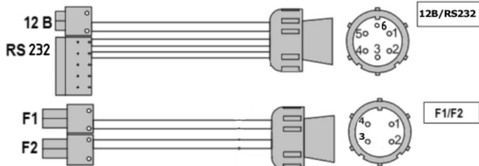
Рисунок Л1 Внутренний шлейф ПРЭМ
