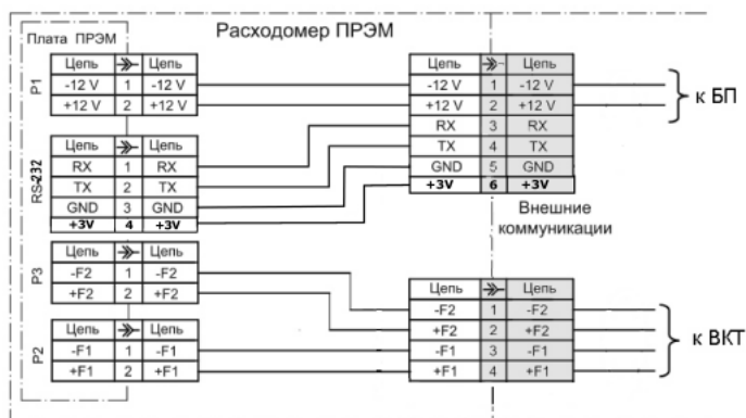
Рисунок Л2 Схема распиновки «выходов» из ПРЭМ
