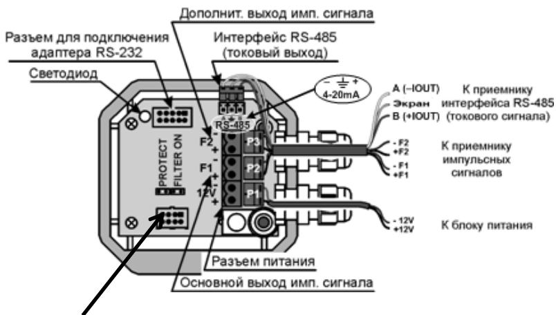
Рисунок М3 Разъём подключения катушек
