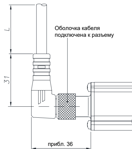
КАБЕЛЬНАЯ СБОРКА С УГЛОВЫМ РАЗЪЕМОМ
