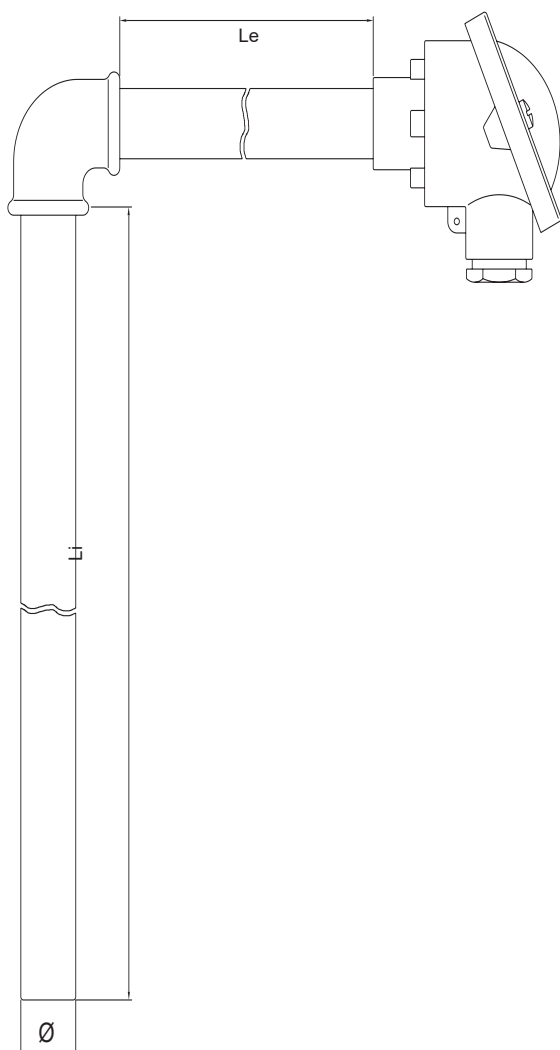
TC10 A с изгибом плеча
