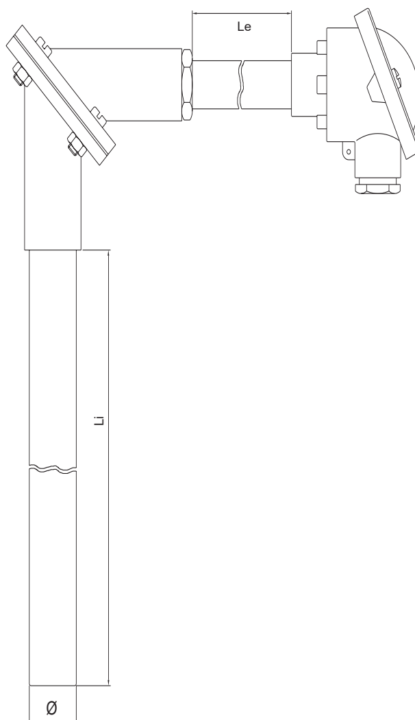
TC10 B с угловым фланцем
