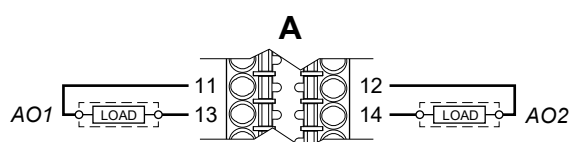
Аналоговые выходы AO1 ... AO8
