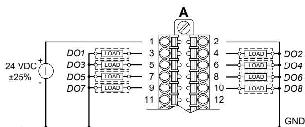
Цифровые выходы DO1 ... DO8
